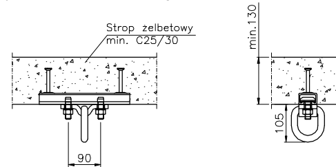
Hak do szybów windowych Jordahl & Pfeifer, model JP01, nośność 20-24 kN.
