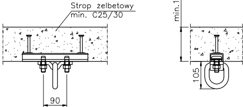
Hak do szybów windowych Jordahl & Pfeifer, model JP01, nośność 20-24 kN.
